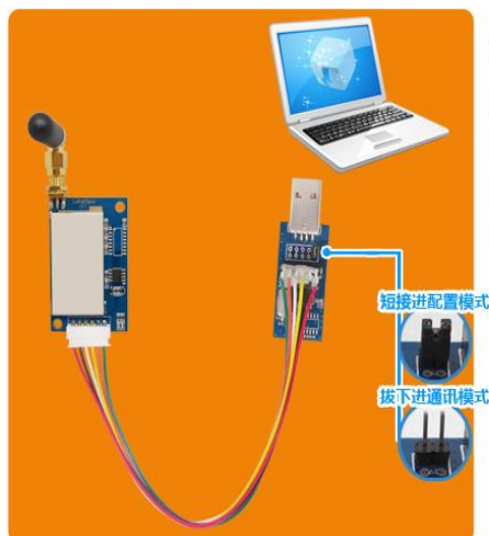
数传模块TTL接口连接示意图
